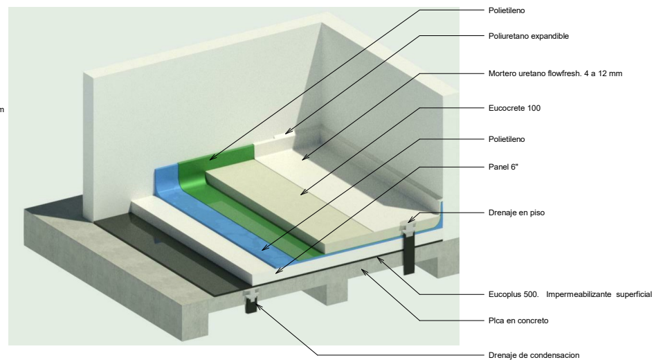
1 Vista 3D 1 : 1
