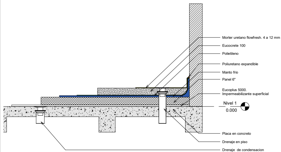
2 Sección 1 1 : 20
