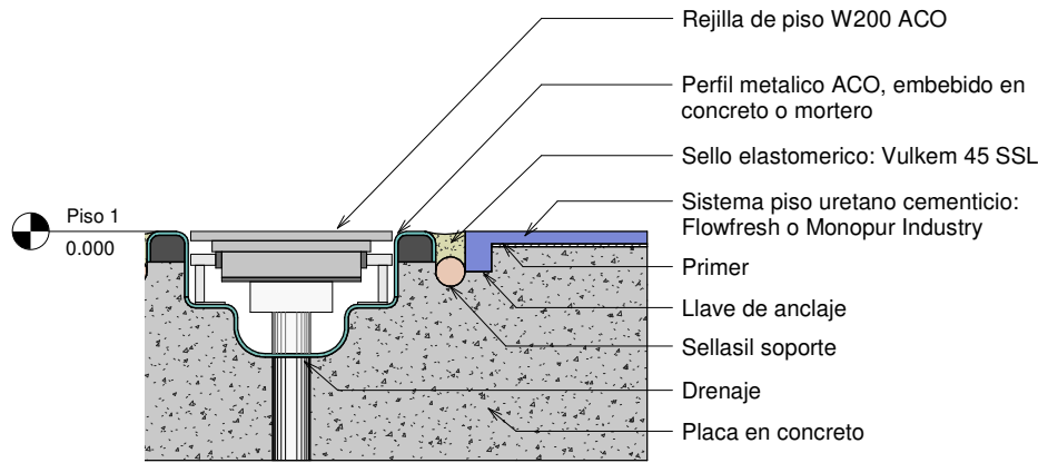
1 Corte 1 1 : 5
