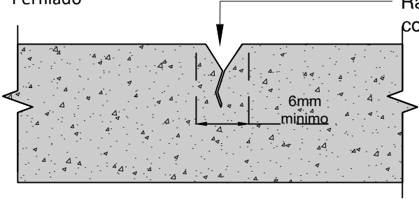
(C) Sellado Mortero de relleno VERTICOAT 1
