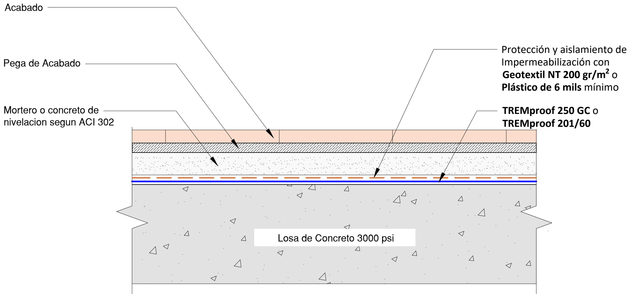
DETALLE SISTEMA TREMPROOF 250 GC
